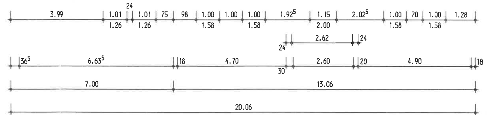
Grundriss Erdgeschoss
